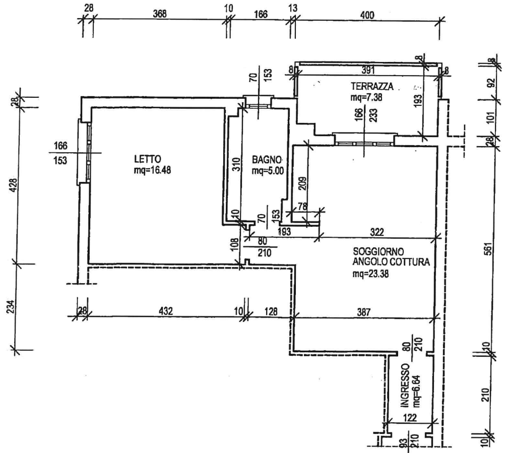
PIANTA APPARTAMENTO - PIANO QUARTO STATO DI FATTO
