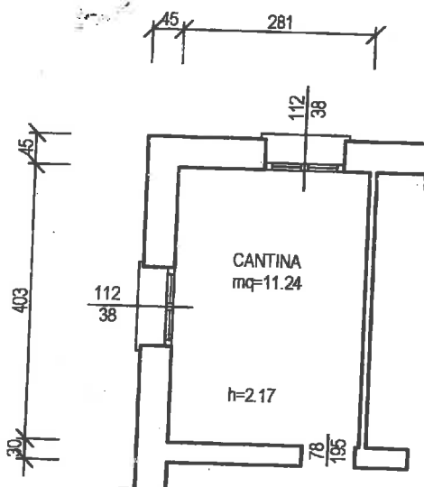
PIANTA CANTINA - PIANO SEMINTERRATO STATO DI FATTO
