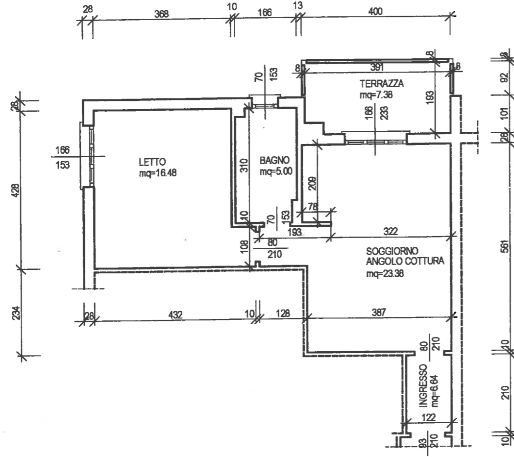
PIANTA APPARTAMENTO PIANO QUARTO
