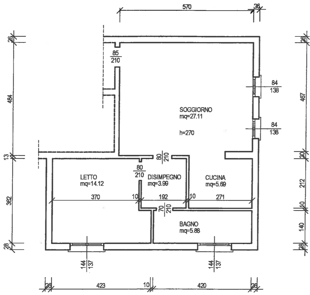
PIANTA APPARTAMENTO PIANO PRIMO
